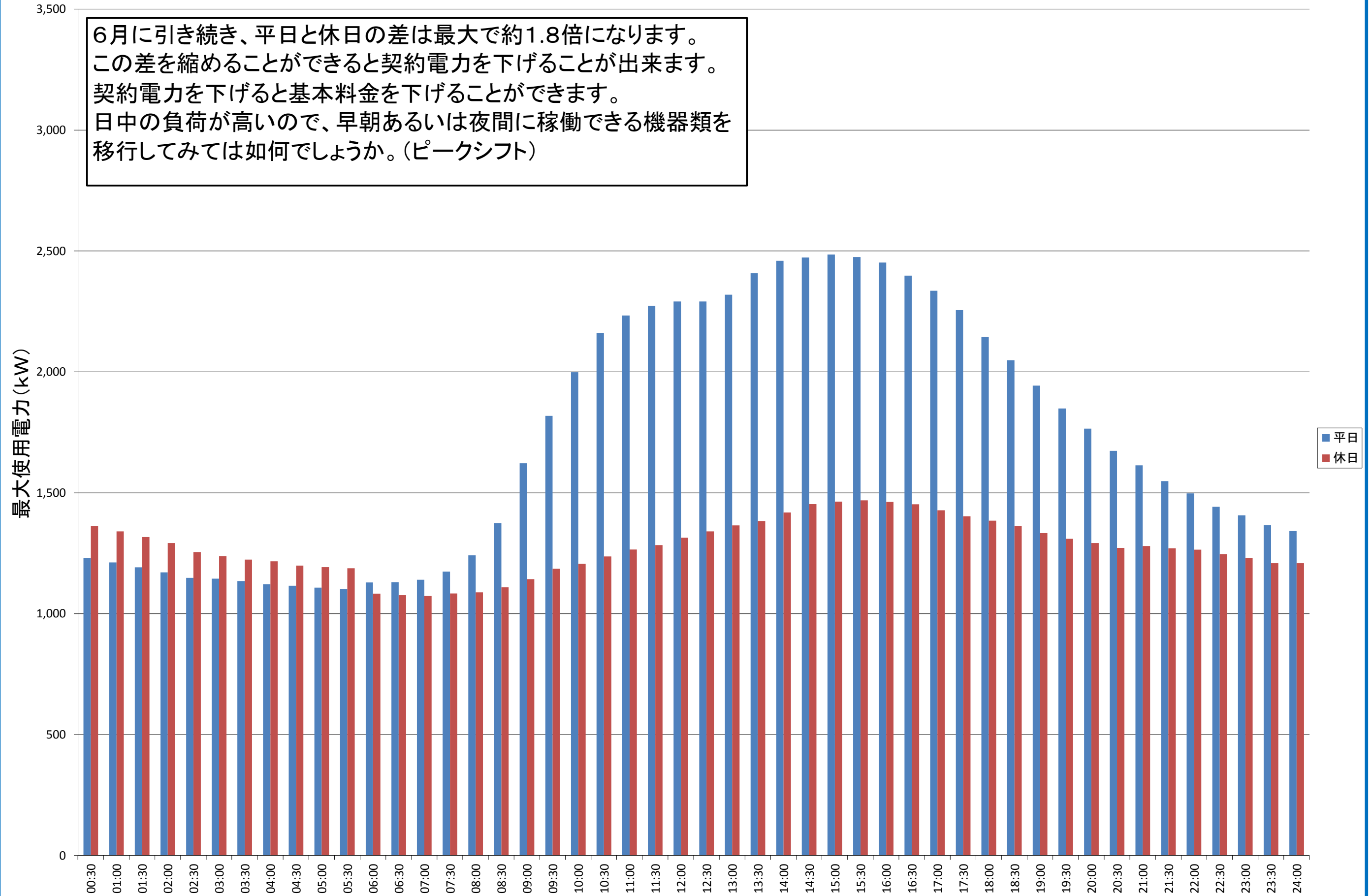
黒髪南キャンパス 7月の時間帯別最大使用電力平均値
