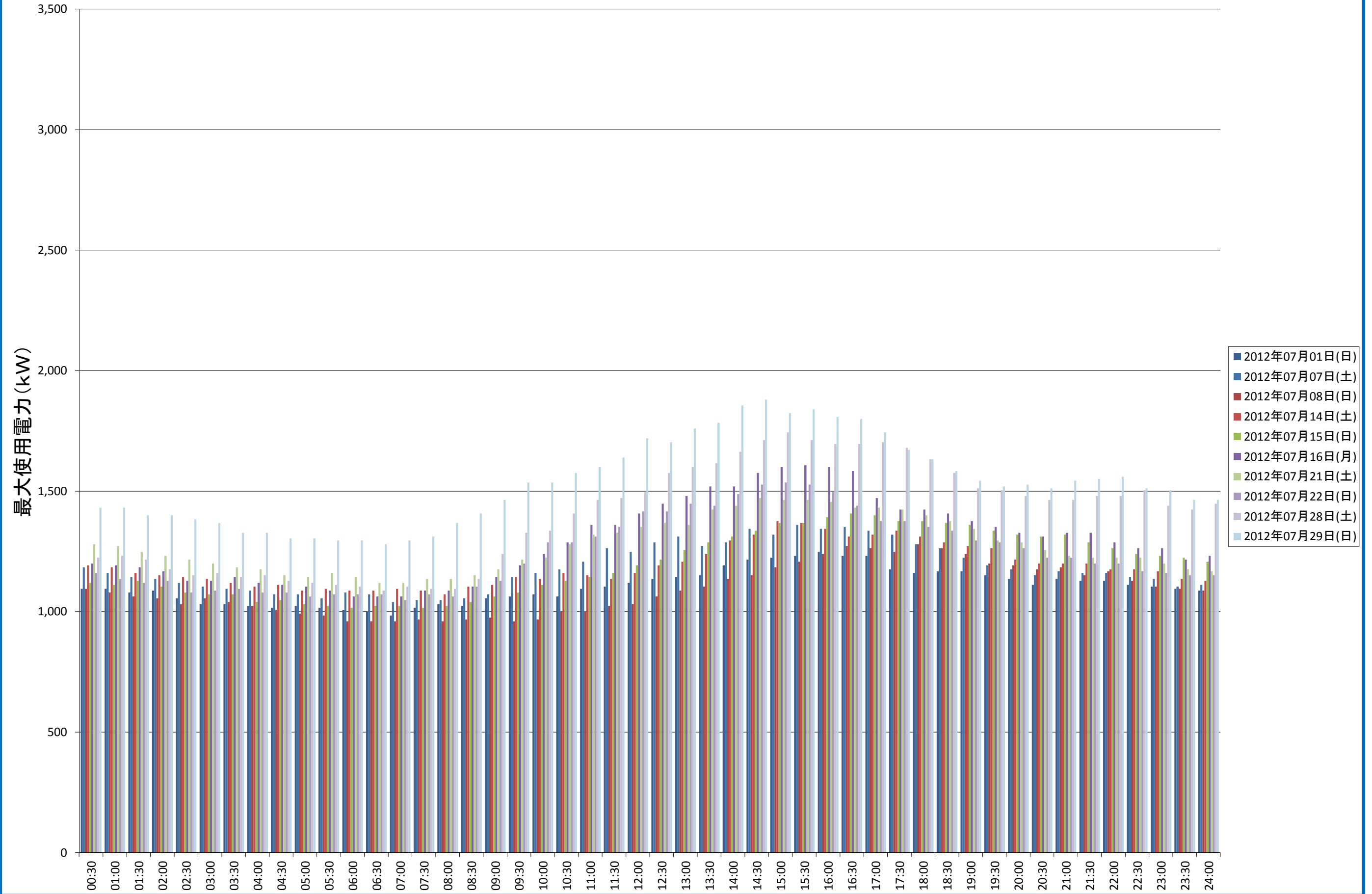
黒髪南キャンパス 7月の時間帯別最大使用電力(土日祝)
