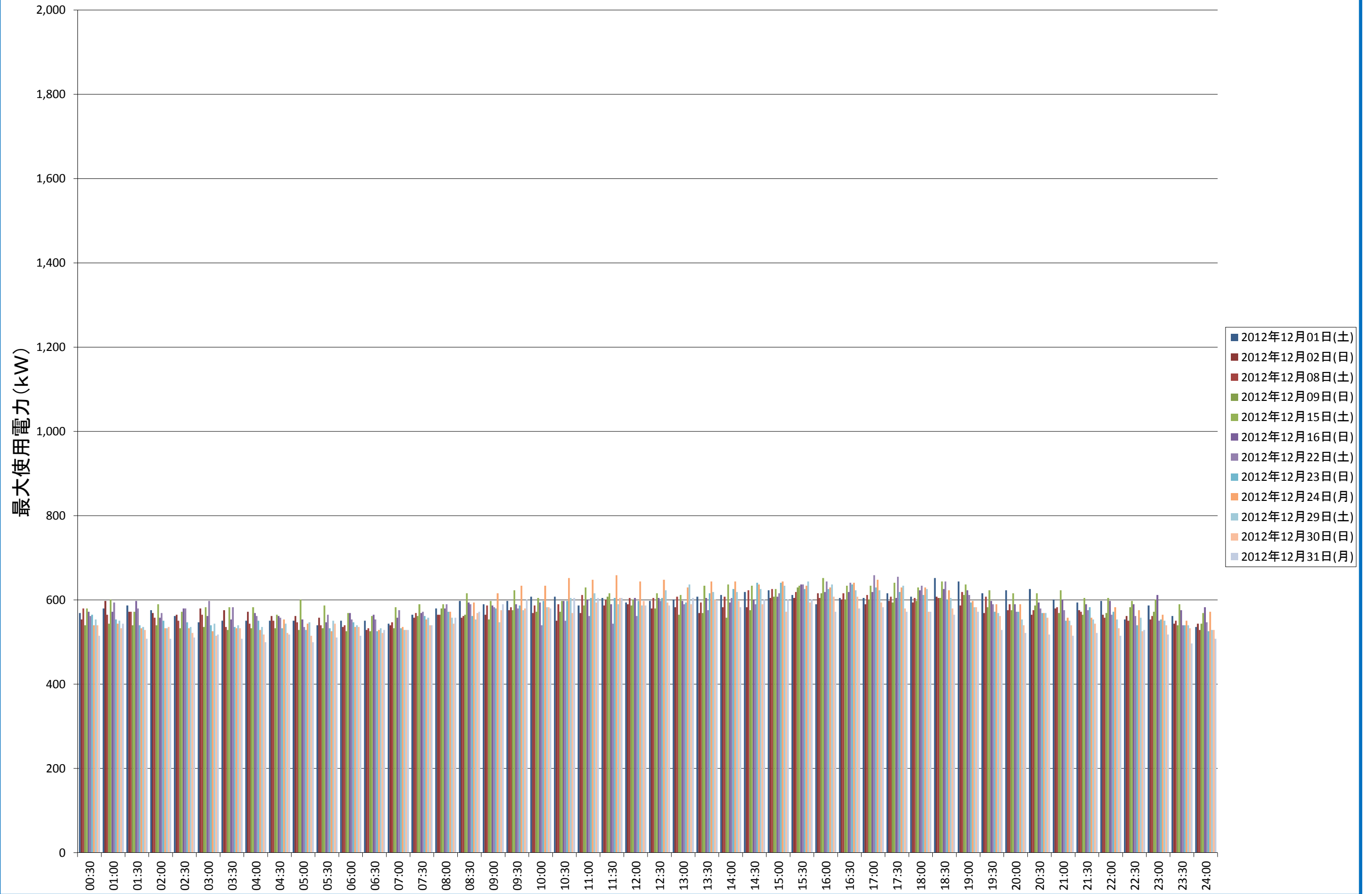
本荘中キャンパス 12月の時間帯別最大使用電力(土日祝)
