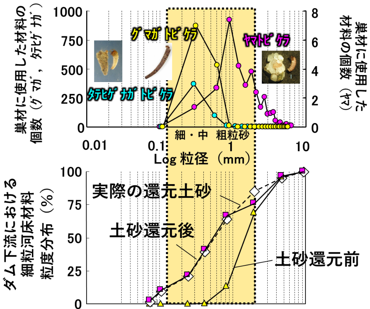
図2 携巣性トビケラの巣材の粒度分布（上）と河床・還元土砂の粒径分布（下）
